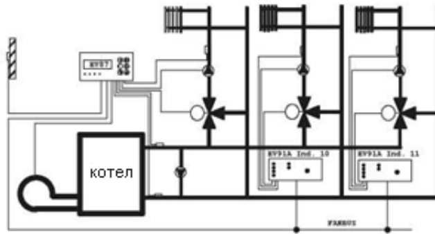
Нагревание 3 областей с одним одноступенчатым котлом (1 EV87 + 2EV91A)
