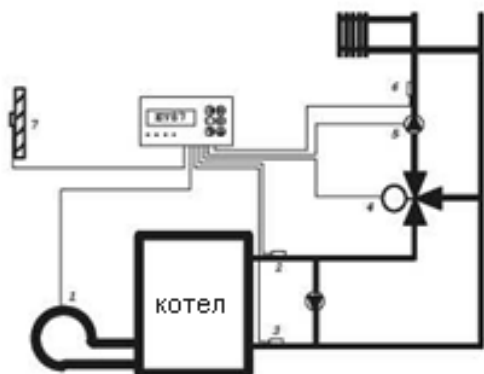
Нагревание 1 области с одним одноступенчатым котлом
