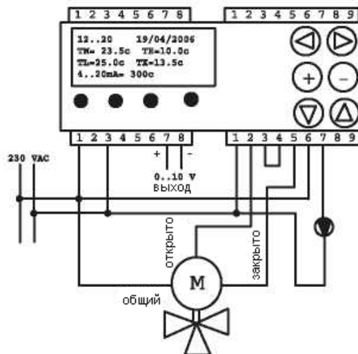
Схема соединения для управления смешивающим клапаном с сервоуправлением питанием 230VAC
