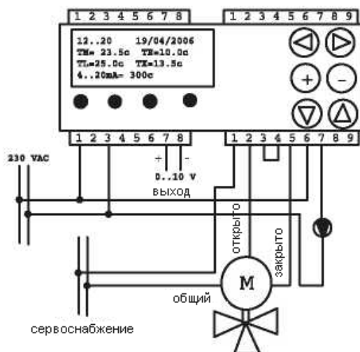
Схема соединения для управления смешивающим клапаном с сервоуправлением питанием другим чем 230VAC
