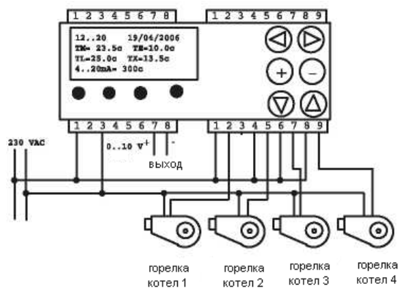
Схема соединения для двухпозиционного регулирования четырех одноступенчатых котлов
