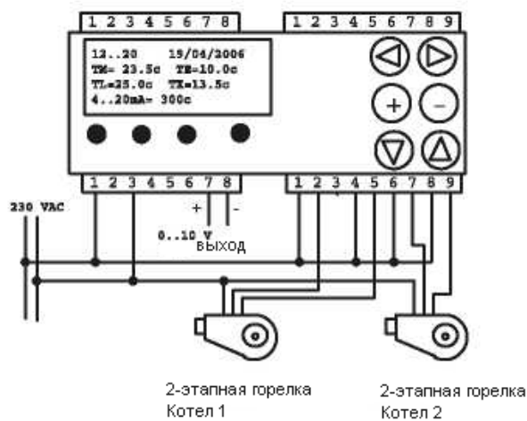
Схема соединения для двухпозиционного регулирования двух двухступенчатых котлов
