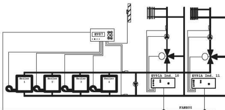
Нагревание 2 областей с четырьмя одноступенчатым котлами в каскаде (1 EV87 2 EV91A)
