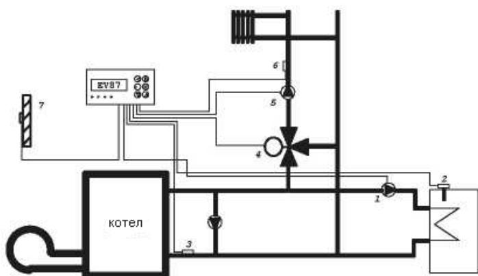
Нагревание 1 области с резервуаром хранения воды для коммунально-бытового водоснабжения
