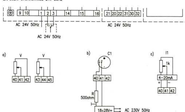
ZAPOJENÍ SVORKOVNICE 24V 50Hz
