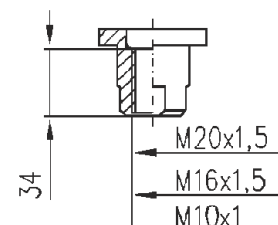
Чертеж муфты
