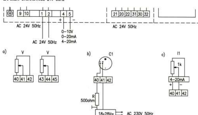
ZAPOJENÍ SVORKOVNICE 24V 50Hz
