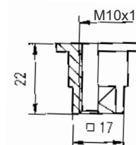
Размеры муфты
